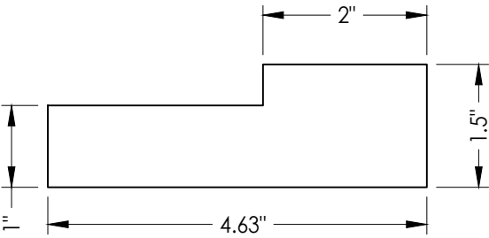
3 WOOD SIDELITE JAMB
