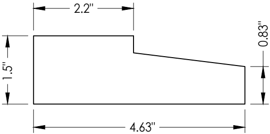
2 WOOD DOOR SILL
